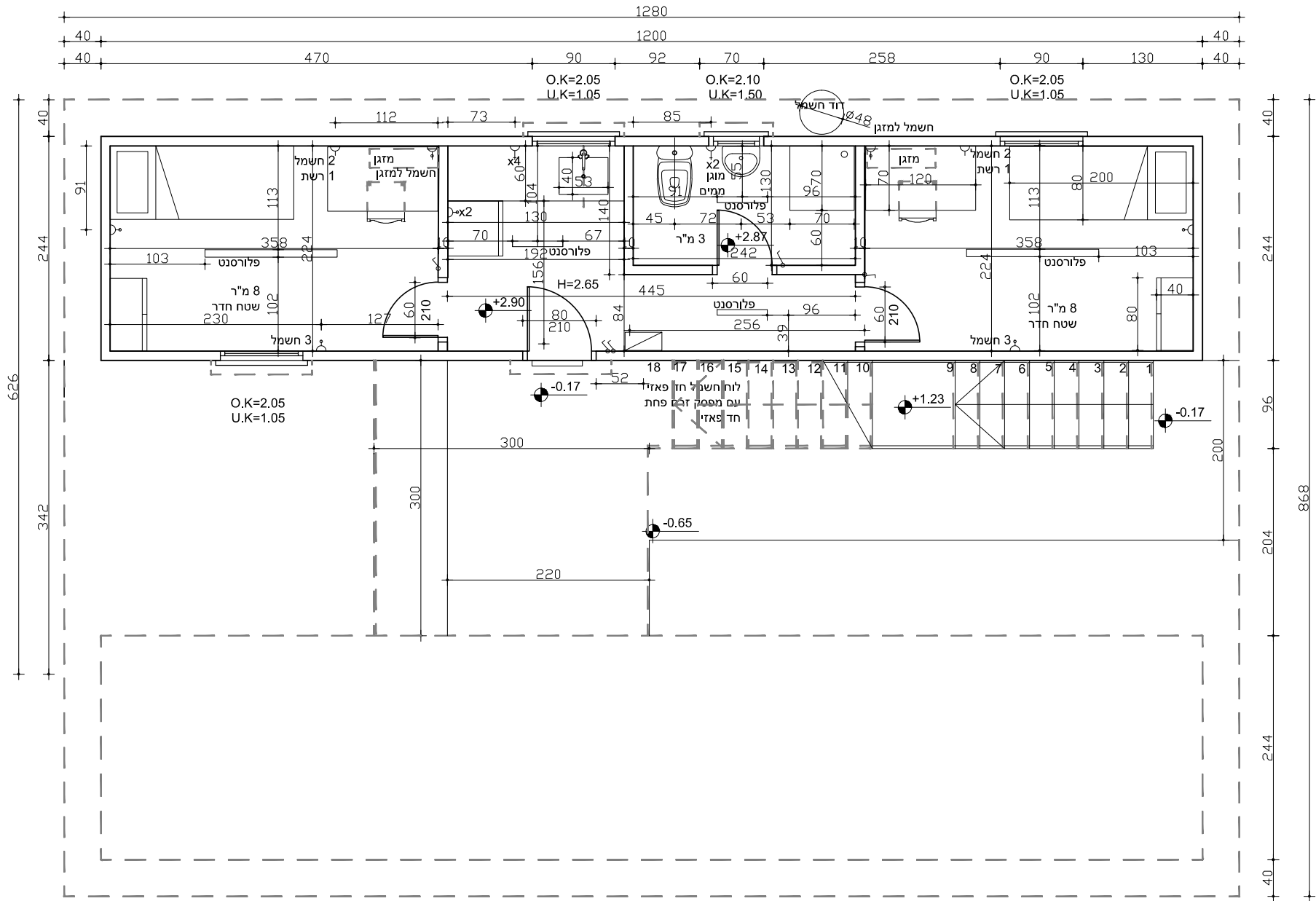
תכנית קרקע 1:60
