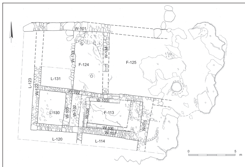
איור 5: האגף הדרומי – תכנית
