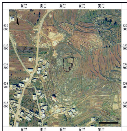
איור 2: תחום האתר ומכלול הבנייה – תצ"א ומפה טופוגרפית
