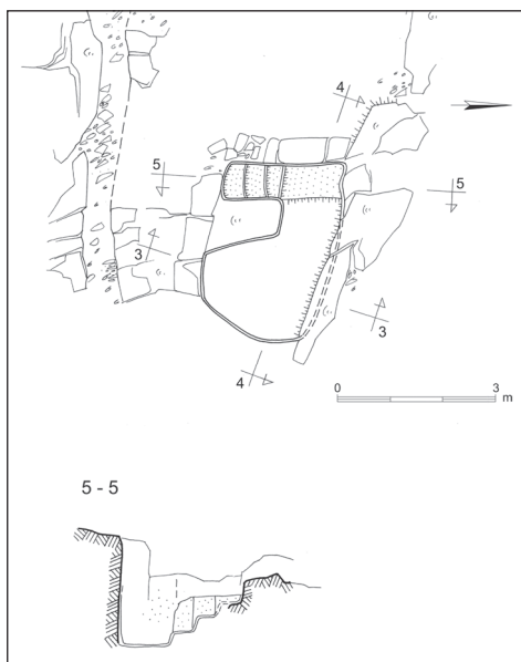
איור 10: המקווה – למעלה: מראה כללי, מבט ממזרח; למטה: תכנית וחתך
