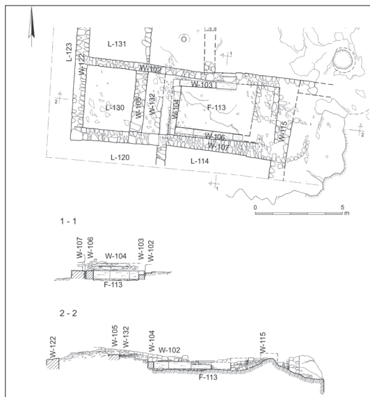
איור 6: מבנה בית הכנסת – תכנית וחתכים
