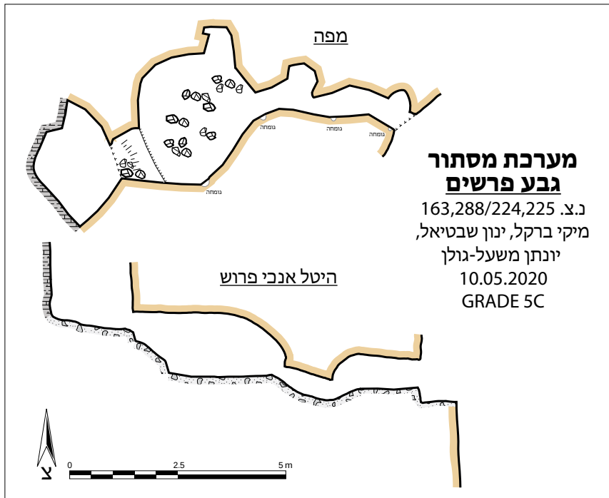
איור 4: מערכת המסתור בגבע - תוכנית וחתך
