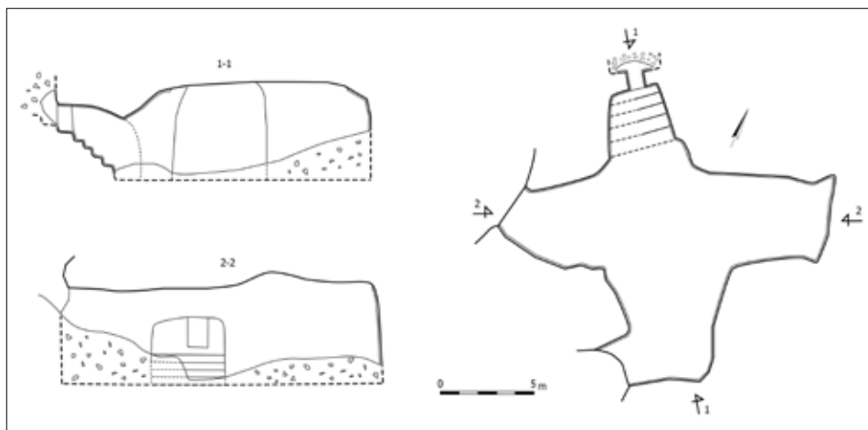
איור 7: בור 3 - תוכנית וחתך
