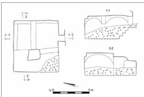
איור 11: מערה 9 - תוכנית וחתכים
