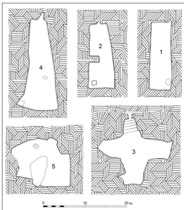
איור 5: תוכניות בורות המים באתר
