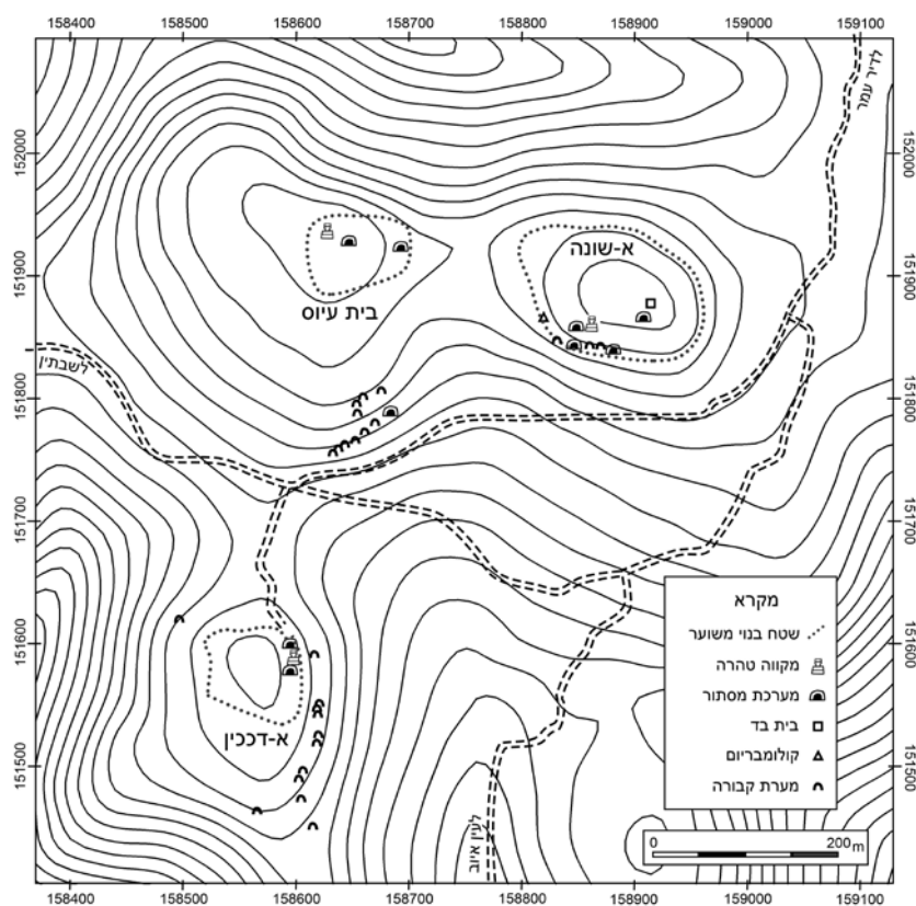
איור 5: ח'רבת א־שונה וסביבותיה - תוכנית השרידים
